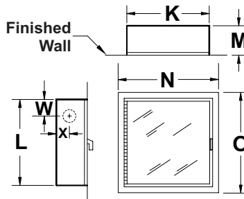
TRIMLESS
