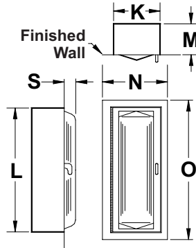
TRIMLESS
